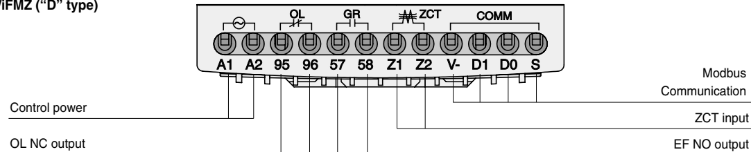
EOCR-i3MZ/iFMZ ("D" type)
