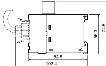
PANEL & DIN RAIL TYPE
