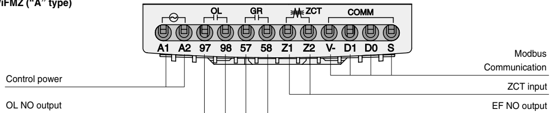
EOCR-i3MZ/iFMZ ("A" type)
