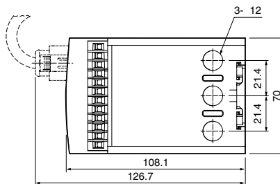
PANEL & DIN RAIL TYPE
